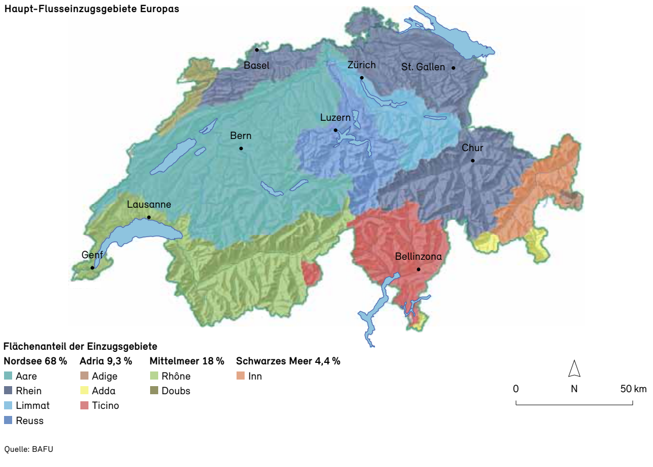
Abbildung 35 Haupt-Flusseinzugsgebiete Europas
